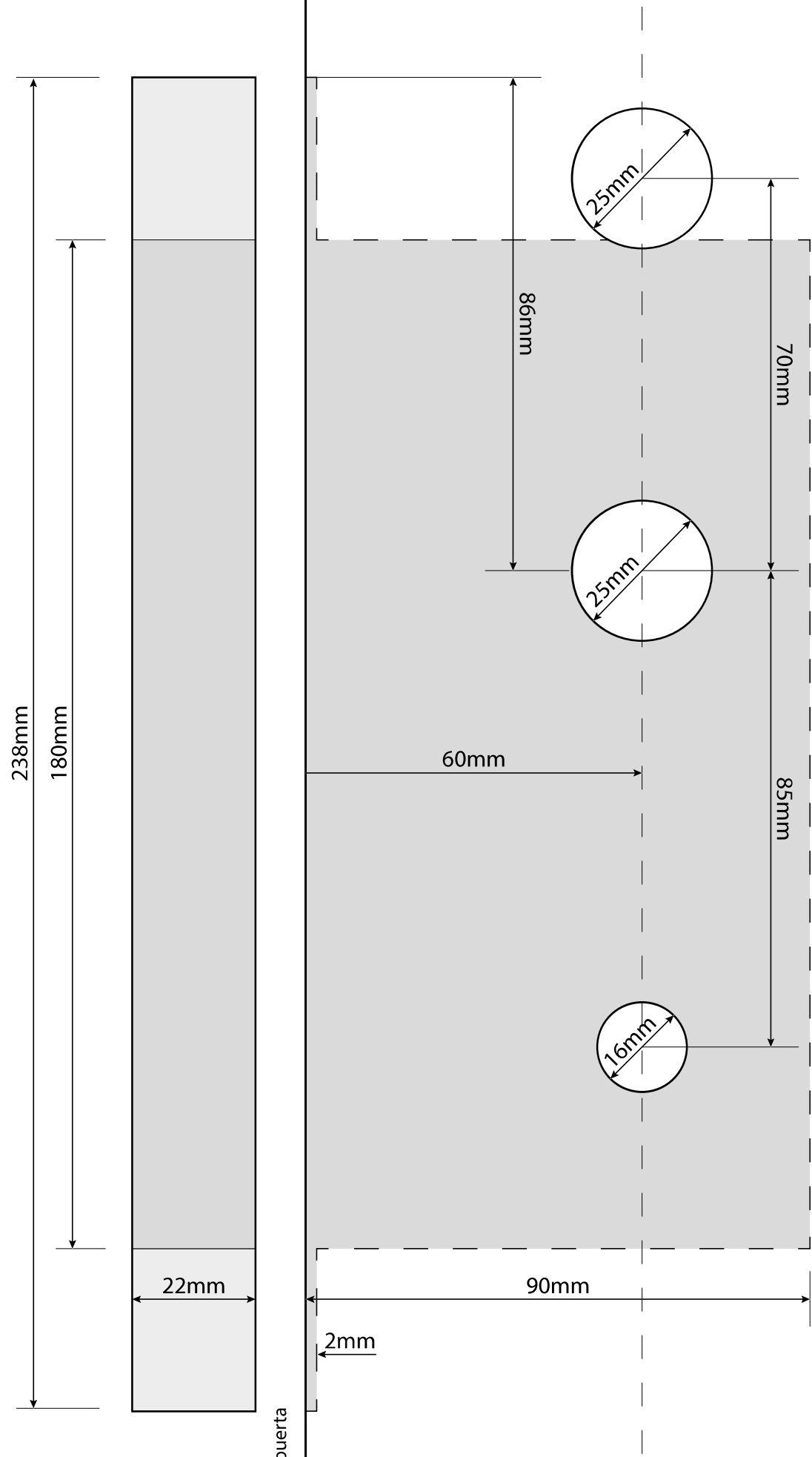
Plantilla de Perforación SHM-H40
